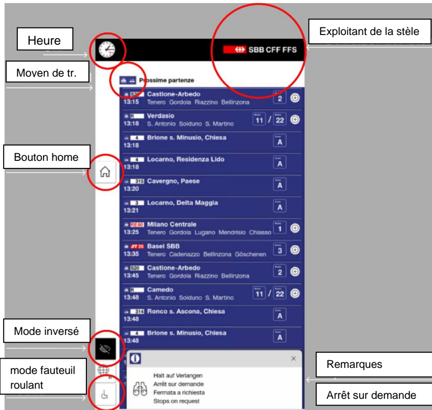
Fig. 280: positionnement des éléments de navigation et des éléments secondaires dans la vue des prochains départs
